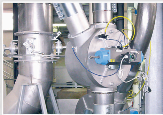
- Válvula diversora em um sistema de tubulação pneumática
